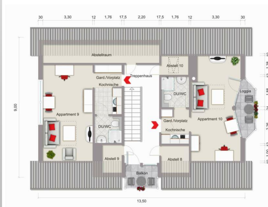
Dachgeschoss
